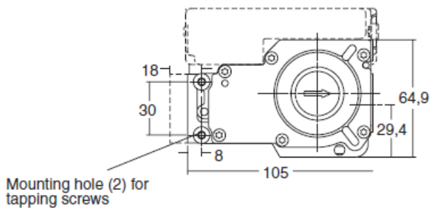
Fig. 1. Dimensions
